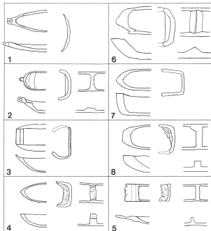
Risbe tipov čolnov Die Zeichnungen der Typen der Kähne
